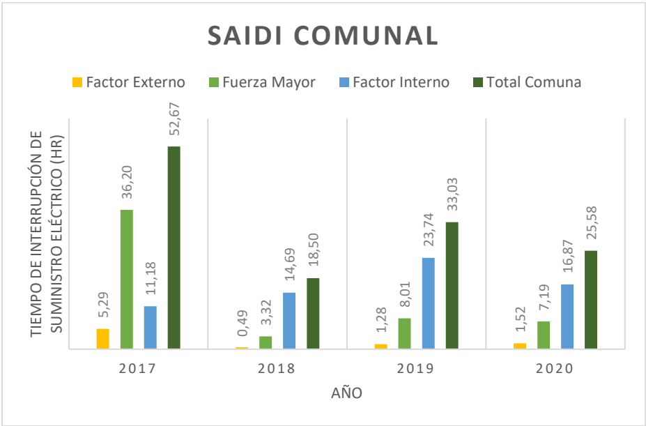
Figura 15: SAIDI comunal. Fuente: Energía abierta.
