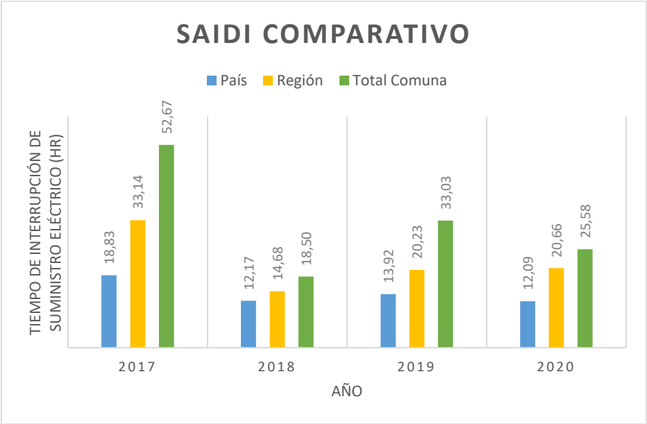
Figura 14: SAIDI comparativo de la comuna. Fuente: Energía abierta.
