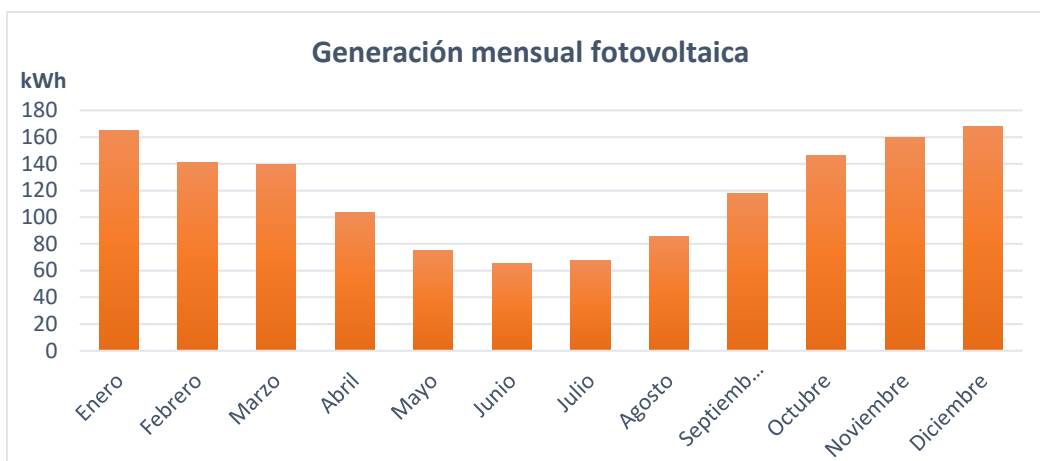
Figura 36: Generación mensual fotovoltaica para un sistema de 1 kW.
