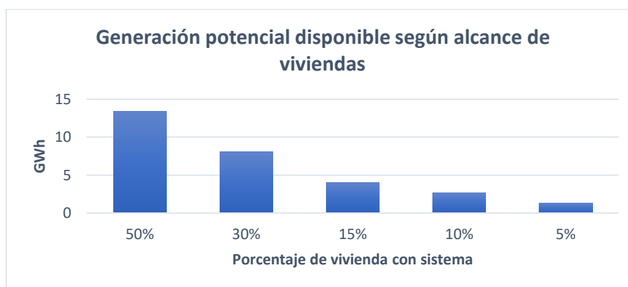
Figura 37: Generación Anual Sistema Inclinado Según Impacto.
