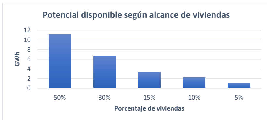
Figura 35: Generación Anual Sistema Inclinado Según Impacto. Fuente: Elaboración propia.
