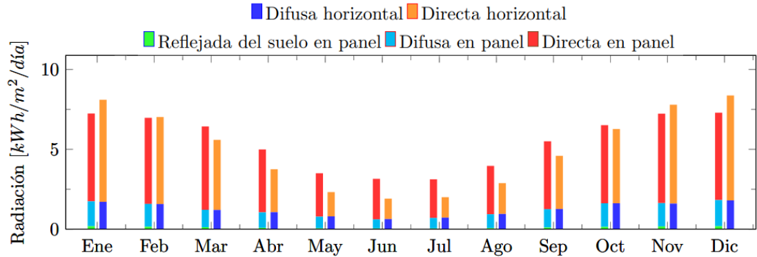
Figura 33: Promedio mensual de la radiación diaria incidente en un plano horizontal y en un plano inclinado, separada en sus componentes directa, difusa y reflejada del suelo.
